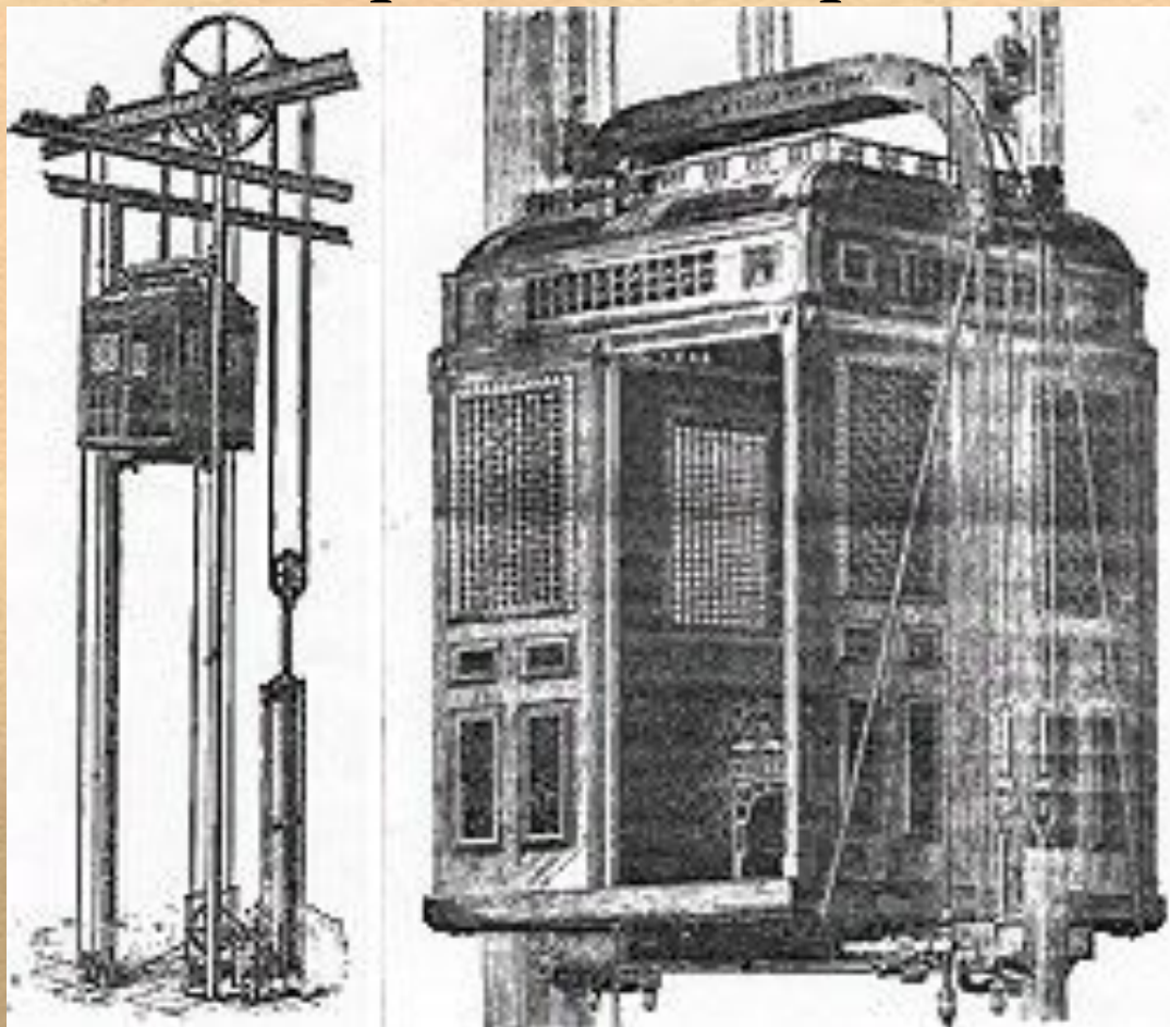
Гидравлический подъемник (лифт), 1793
