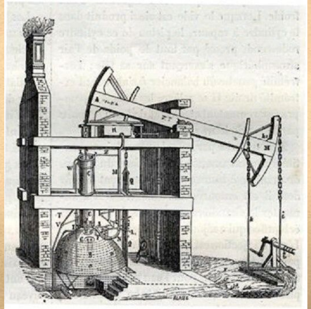
Паровой насос, 1705
