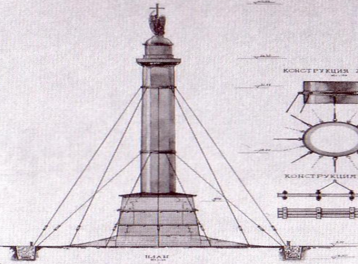
СХЕМА РАСПОЛОЖЕНИЯ АНКЕРОВ И ВАЛТ
