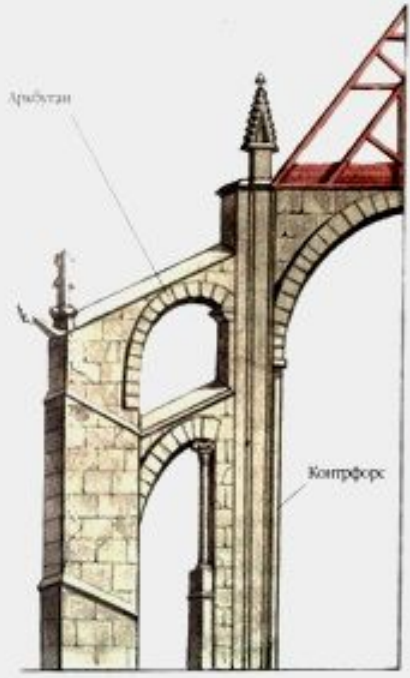
Система арибутов и контрфорсов.
