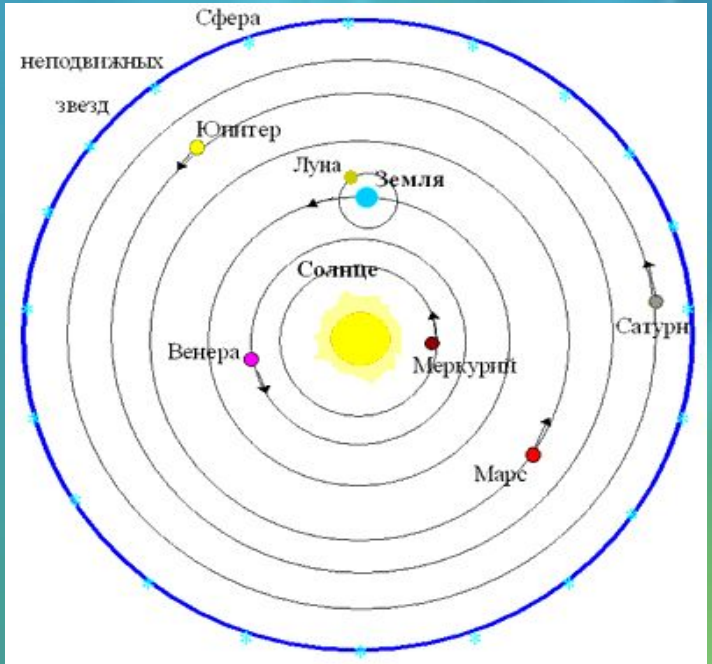
Гелиоцентрическая система
