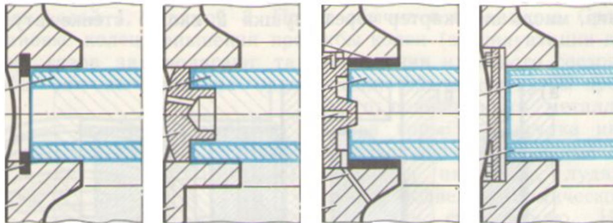
Поршневые пальцы и их крепления
