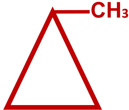
метилциклопропа н
