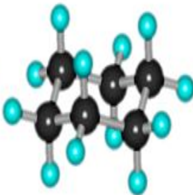
Циклогексан
