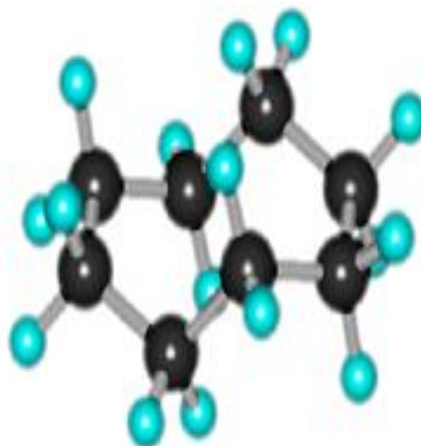
Циклооктан
