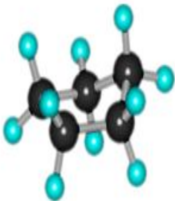
Циклопентан
