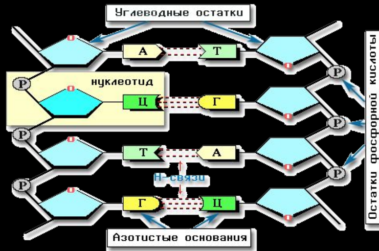
Комплементарность цепей в ДНК
