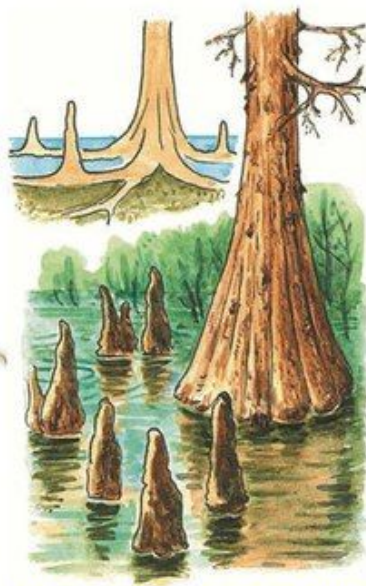
Дыхательные корни
