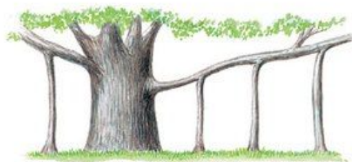
Столбовидные корни
