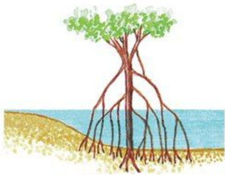
Ходульные корни
