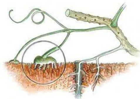
Присасывательные корни
