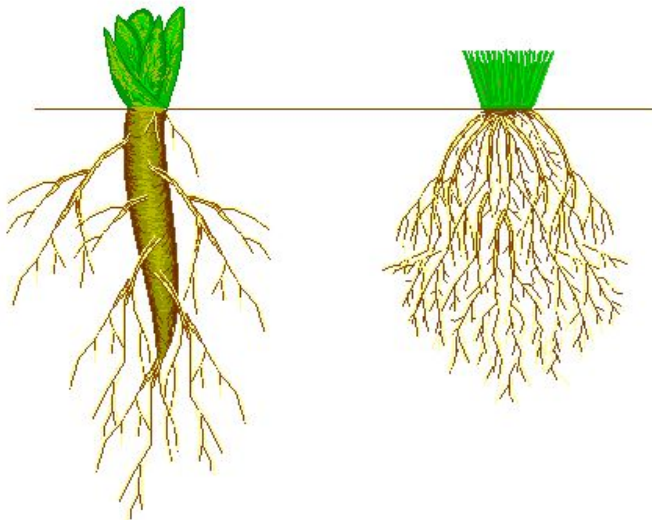
стержневая
