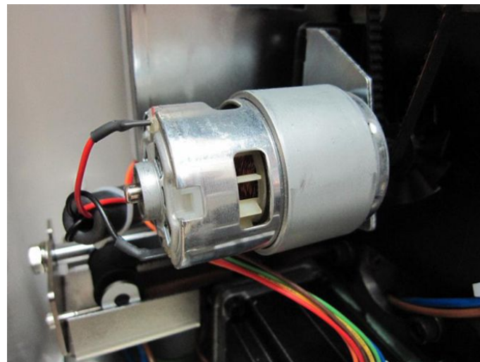
Нарру HCH-701-30, Brother PR – 650/1000, бытового мотор)
