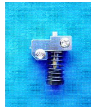
Боринговое устройство
