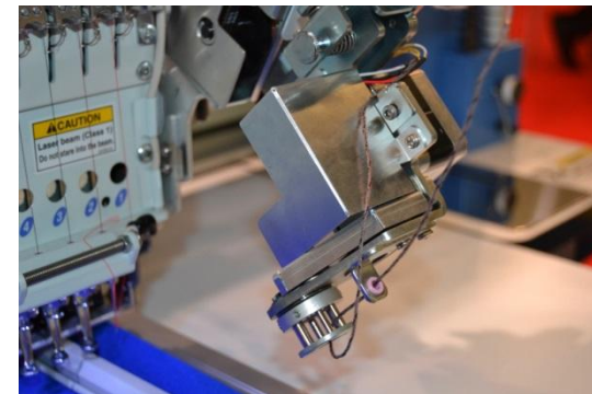
Приспособление для вышивки шнуром
