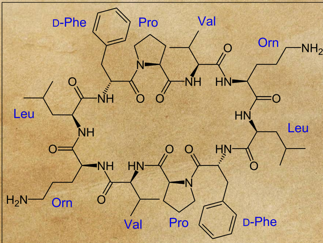
Структурная формула Грамицидина С
