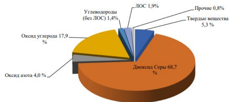
Рисунок 1.31 Состав выбросов загрязняющих веществ от стационарных источников
