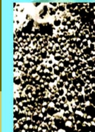
Подводная фотография покрова железо-марганцевых конкреций на дне Тихого океана (глубина 5400м)
