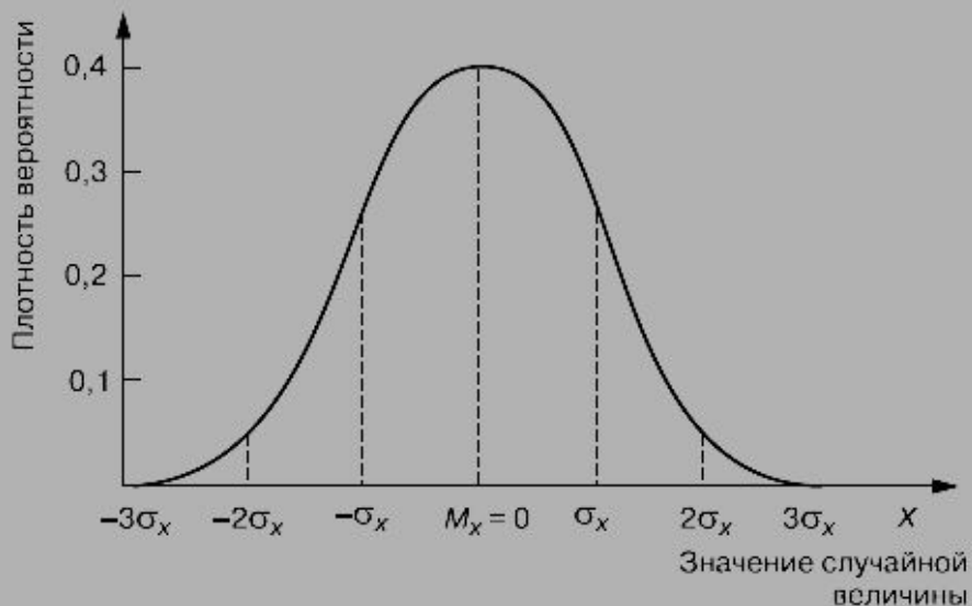
Плотность вероятности нормального распределения
