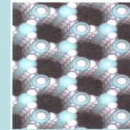
Ячейки из 912 молекул
