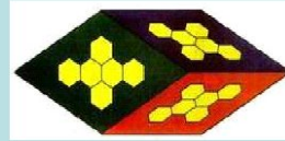
Кластерная модель структурированной воды
