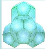
Модель «кванта воды» из 57-и молекул
