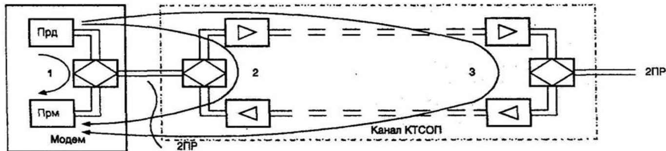
б) с путями прохождения эхо-сигналов (1, 2, 3)
