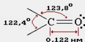
Геометрия карбонильной группы
