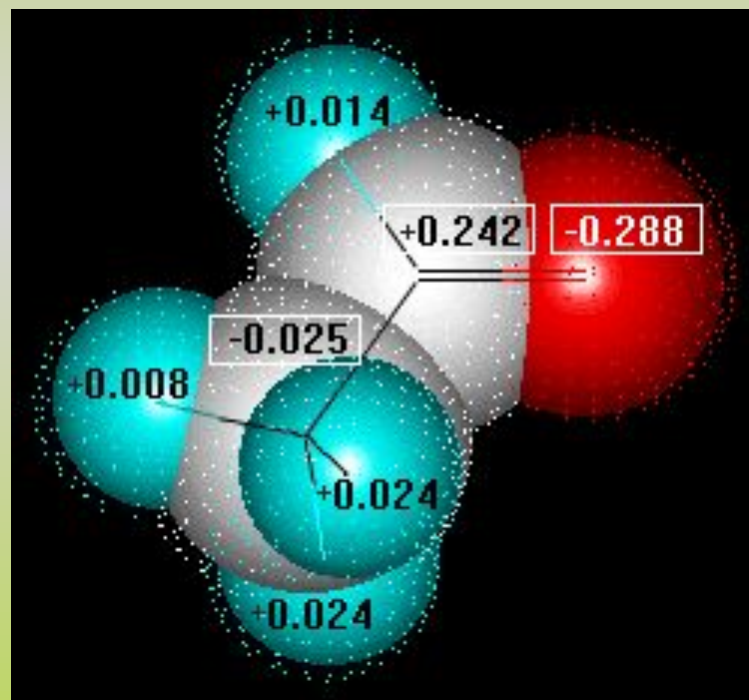
Геометрия карбонильной группы
