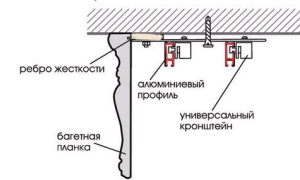
потолочное крепление
