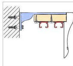
К стене, фанера
