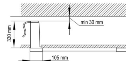
Установка в полый потолок
