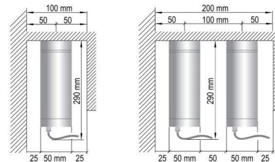
Монтаж в нишу
