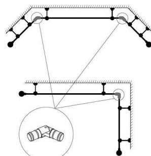
Шарнирный элемент
