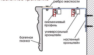
настенное крепление
