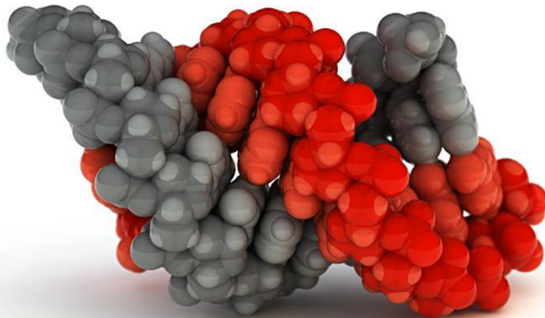
A-DNA
