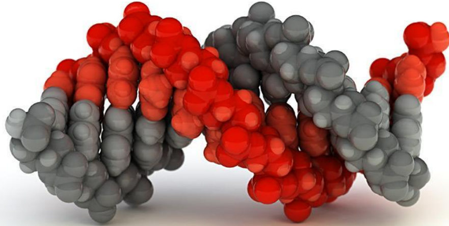
B-DNA
