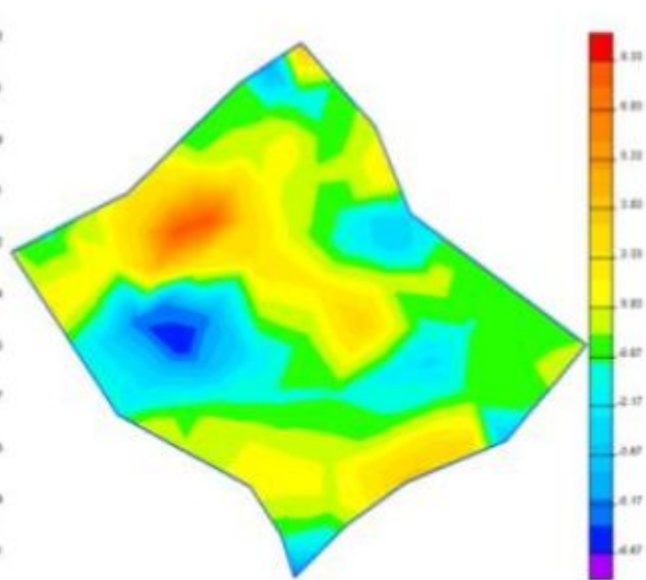
Рис. 10. Деформация \epsilon_{xx} ( 10^{-5} )
