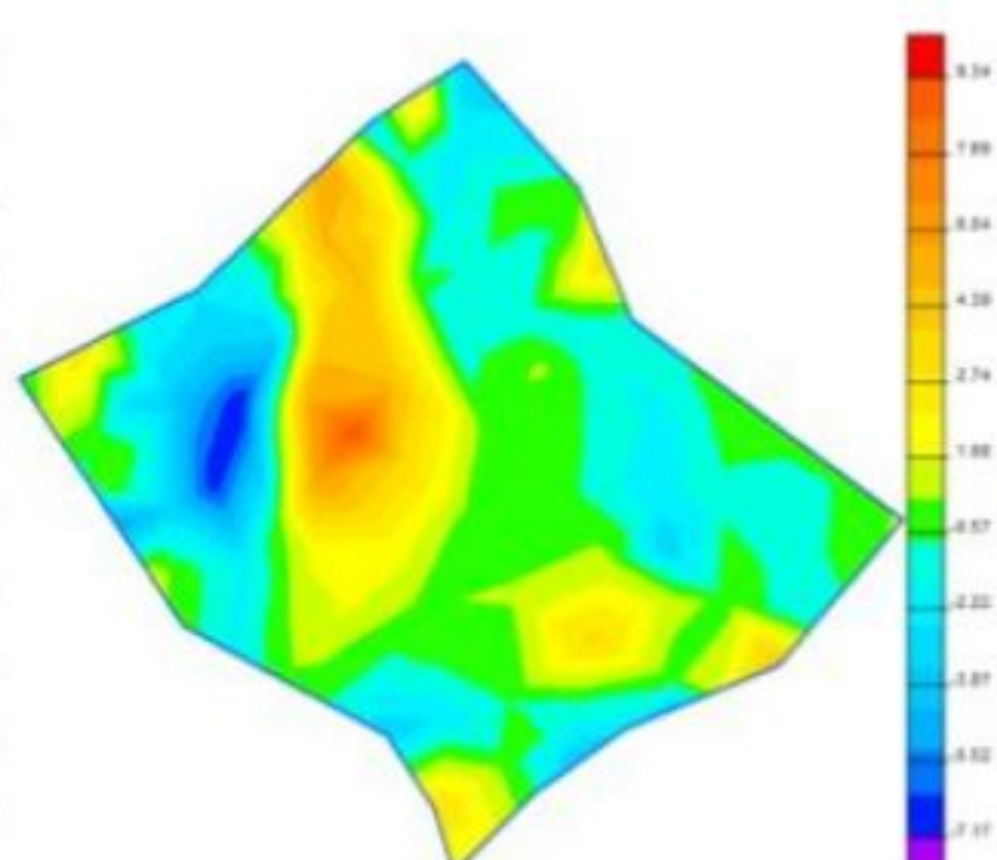
Рис. 12. Деформация \gamma_{xy} ( 10^{-5} )
