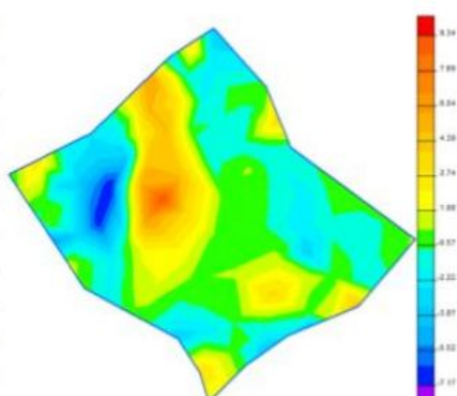
Рис. 12. Деформация \gamma_{xy} ( 10^{-5} )
