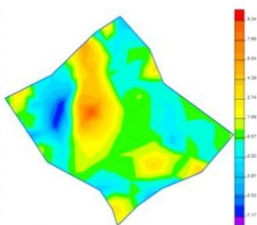
Рис. 12. Деформация \gamma_{xy} ( 10^{-5} )
