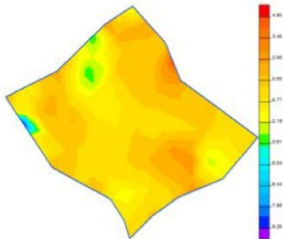
Рис. 11. Деформация \epsilon_{yy} ( 10^{-5} )
