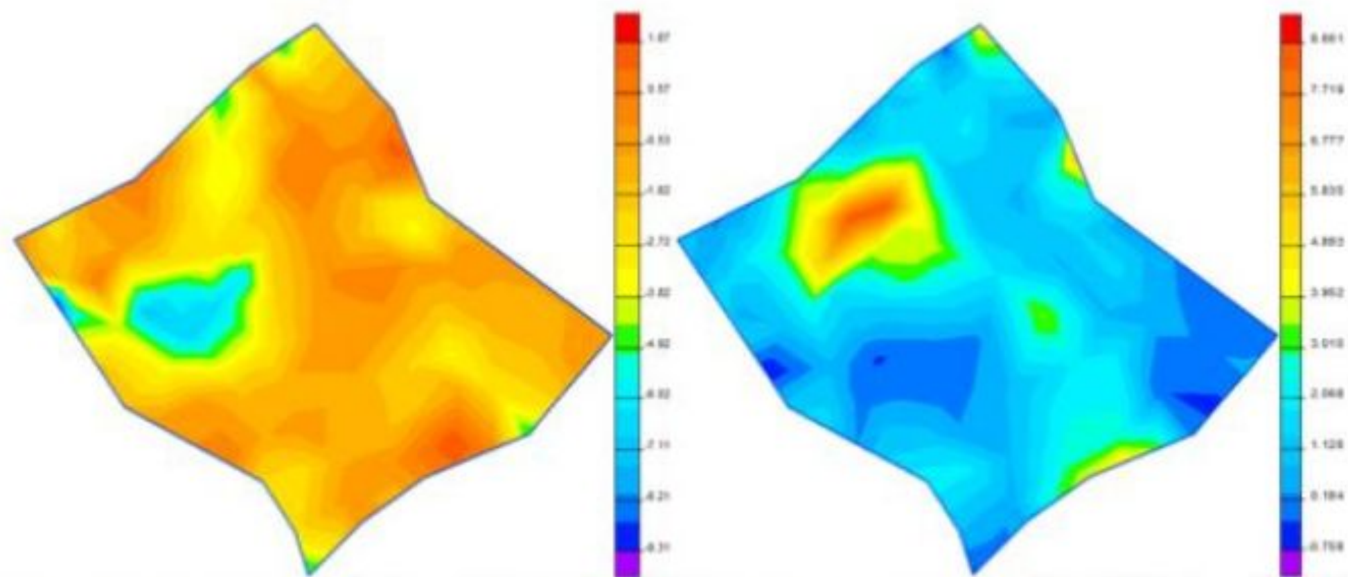
Рис. 13. Главная деформация \varepsilon_1 ( 10^{-5} ) Рис. 14. Главная деформация \varepsilon_2 ( 10^{-5} )
