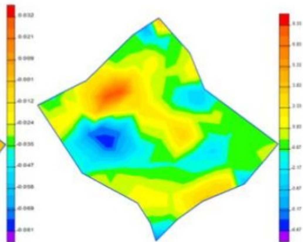
Рис. 10. Деформация \epsilon_{xx} ( 10^{-5} )
