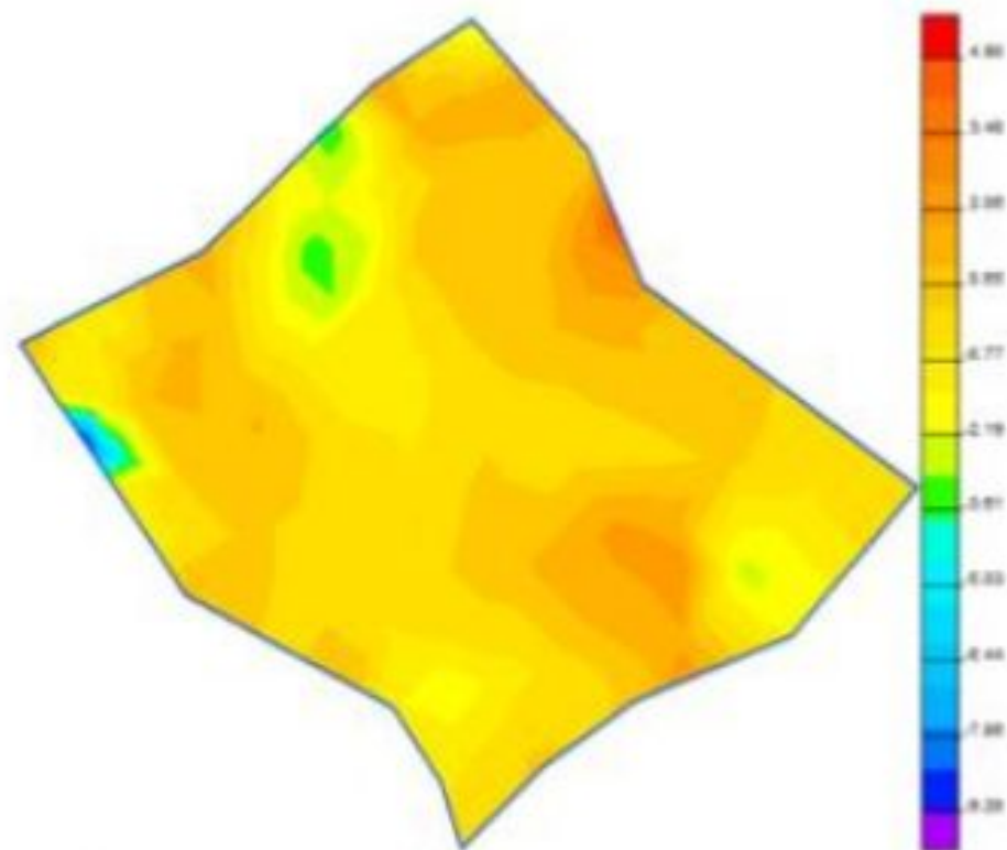
Рис. 11. Деформация \epsilon_{yy} ( 10^{-5} )
