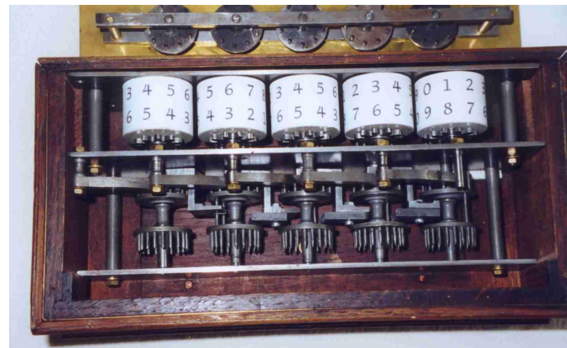
«Паскалина»
