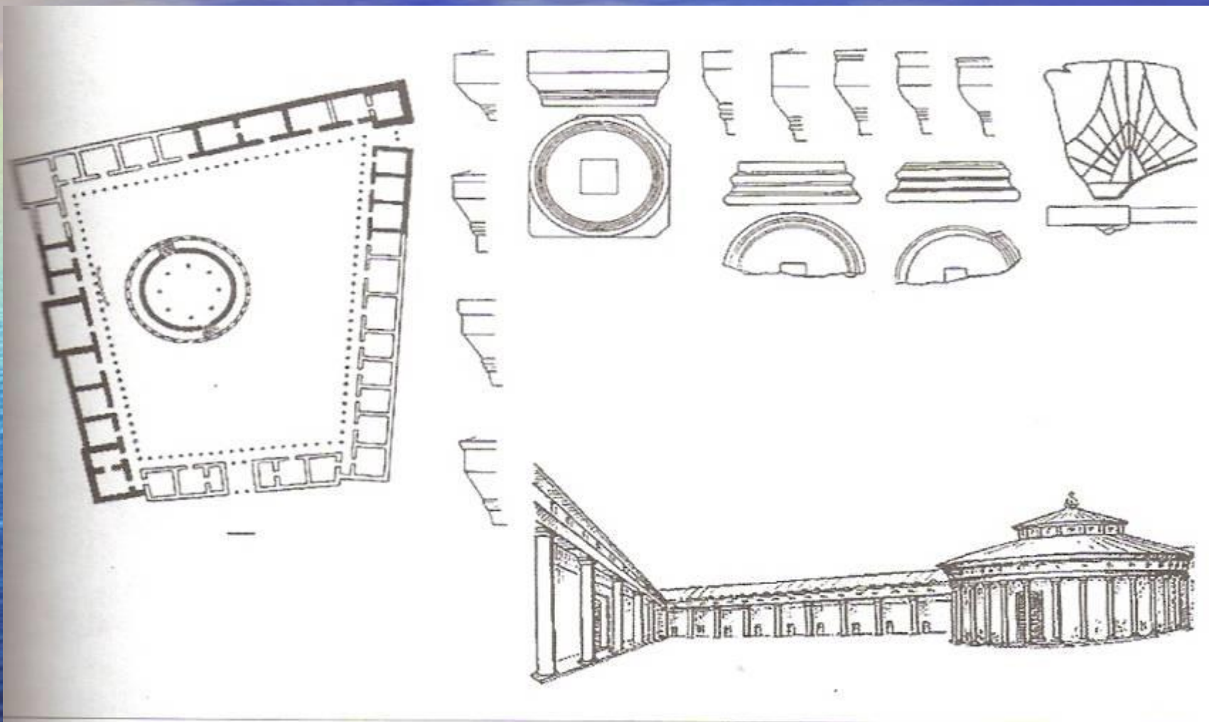
Таманский толос. План и реконструкция
