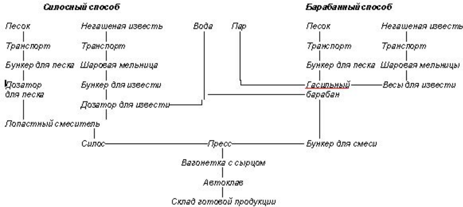
Рис. 2. Технологическая схема производства силикатного кирпича силосным и барабанным способами.
