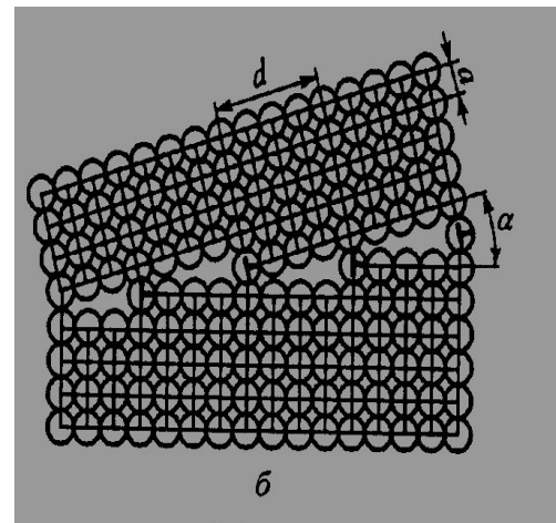
Схема строения малоугловых границ
