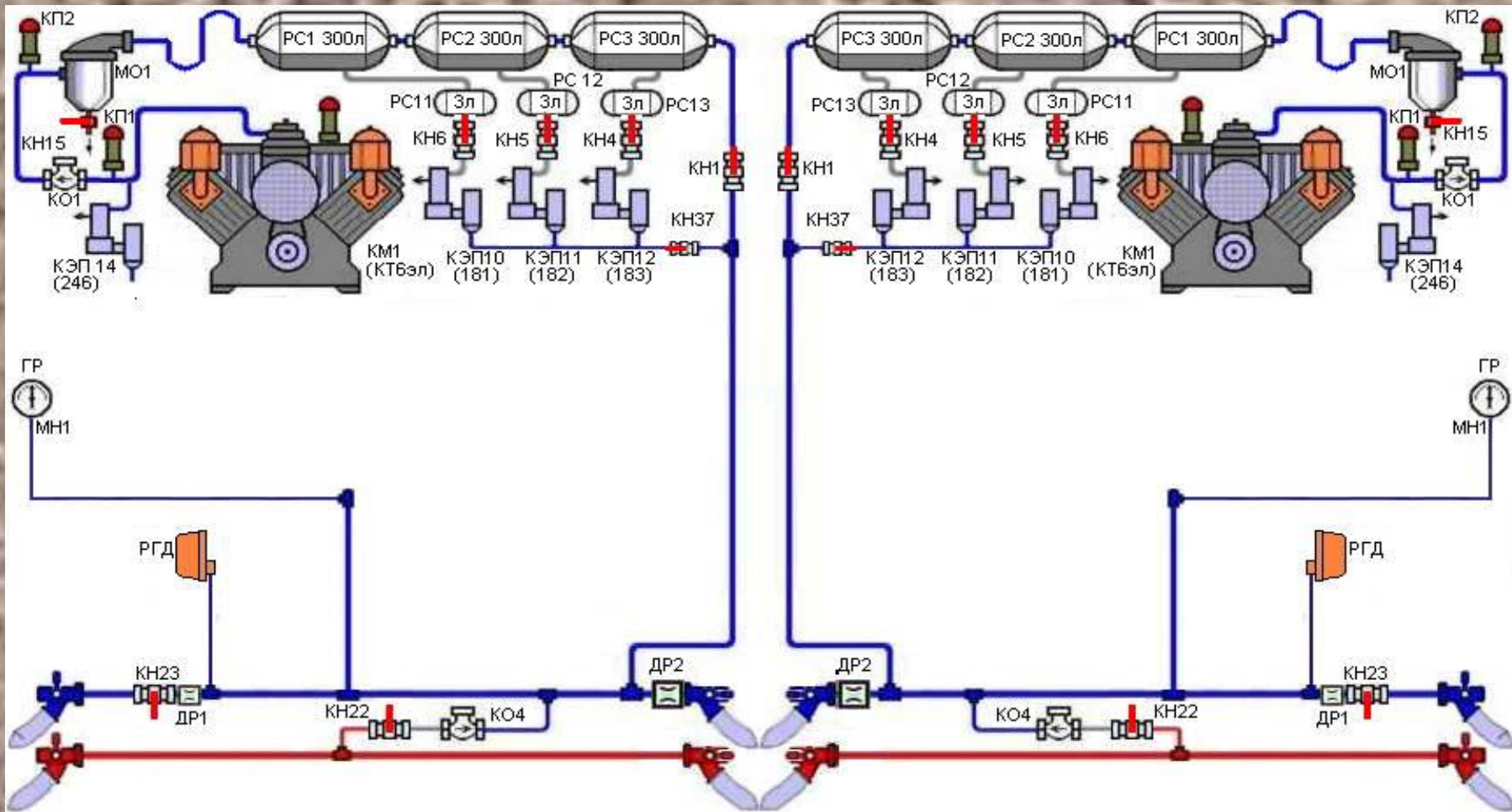
Система питания электровоза сжатым воздухом
