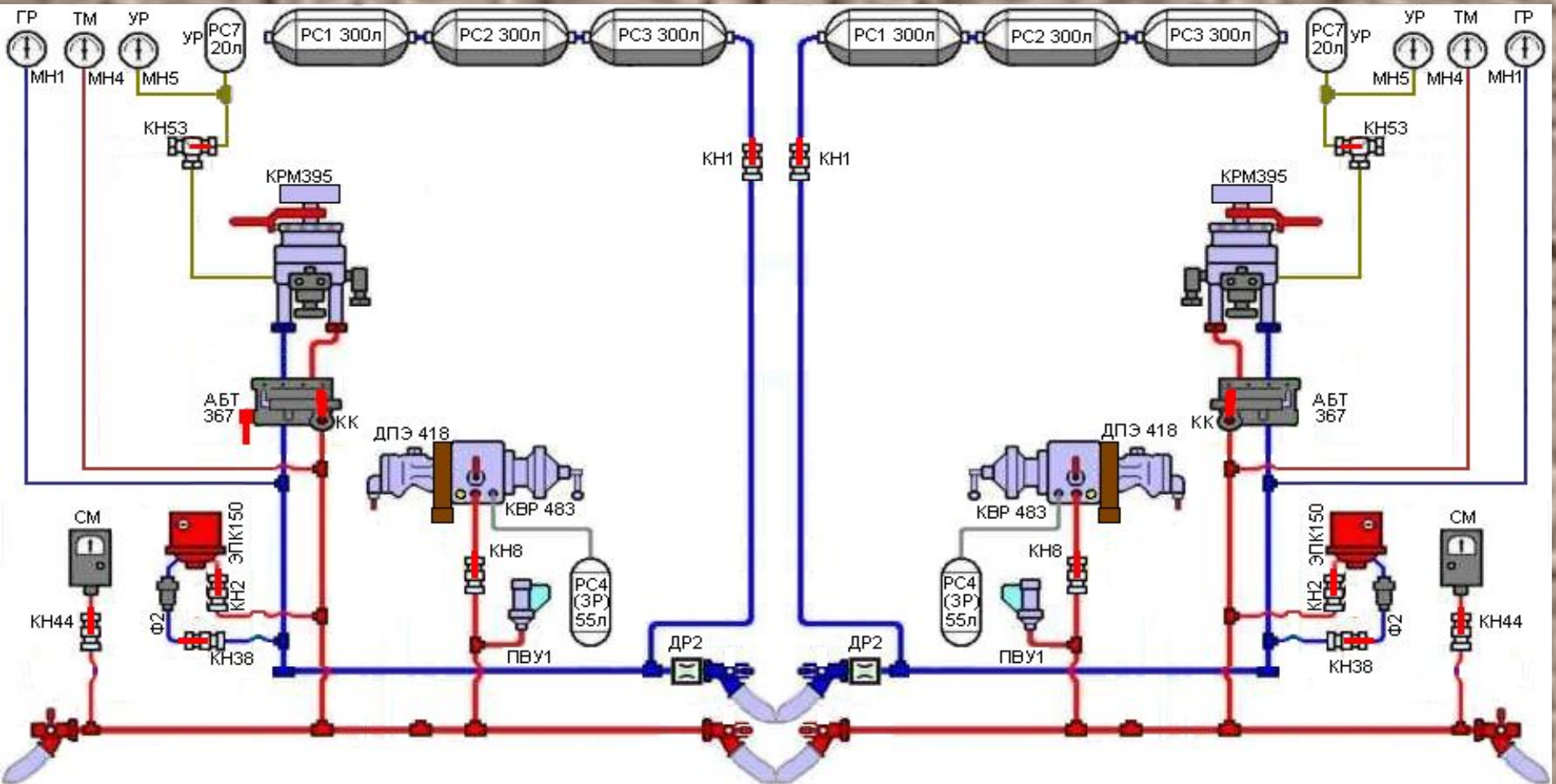
Система зарядки запасных резервуаров
