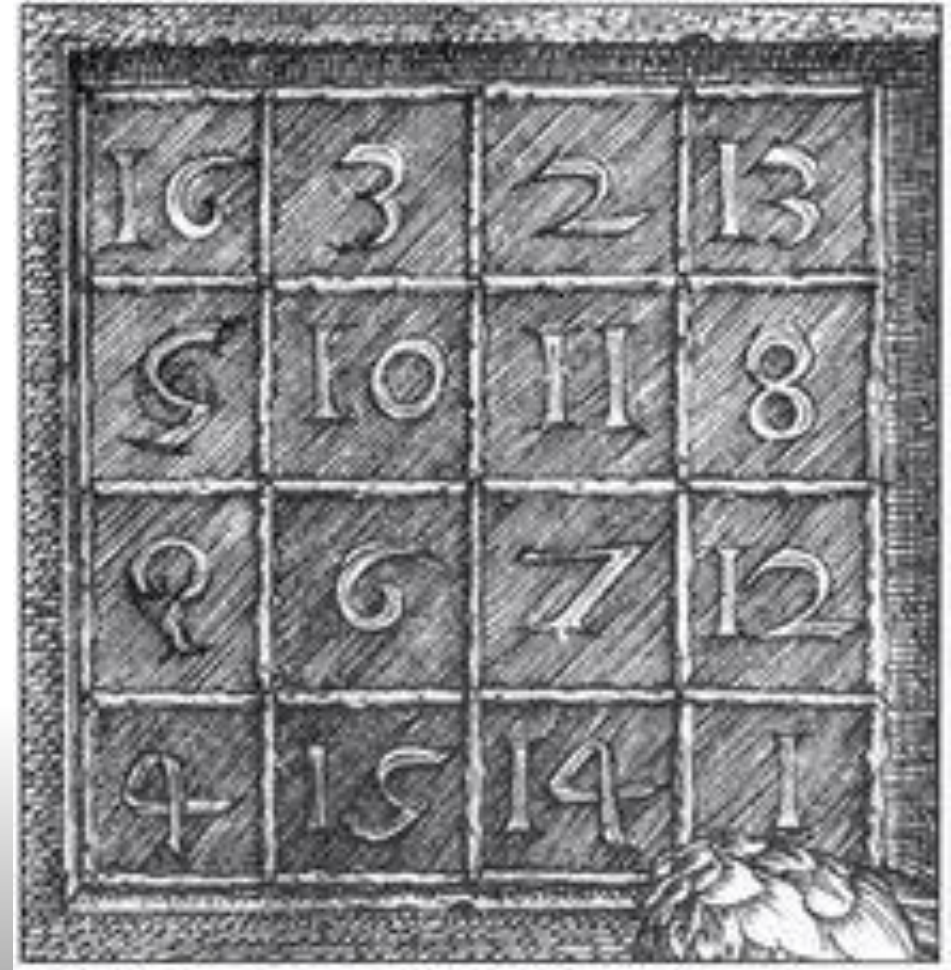
Магический квадрат на гравюре Дюрера «Меланхолия»
