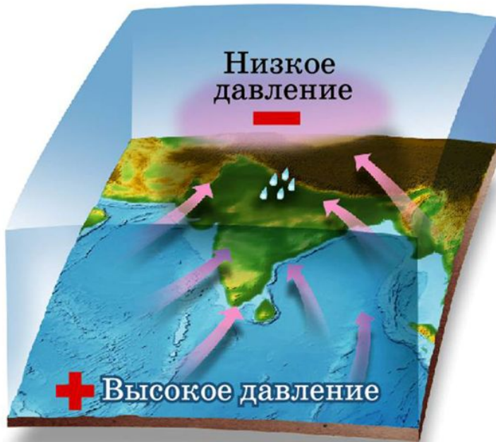
Летний муссон
