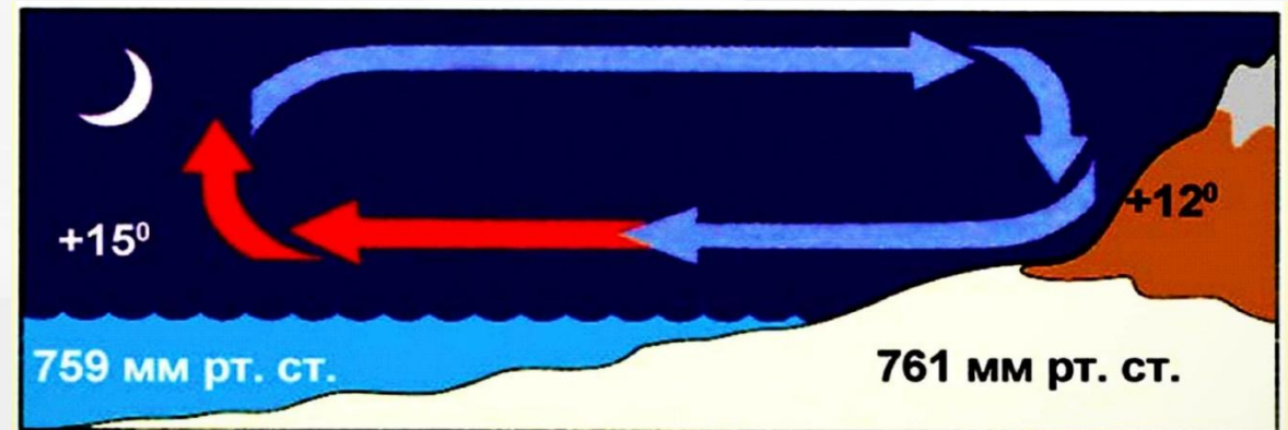
Ночной бриз
