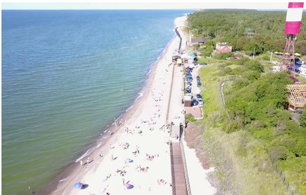
Балтийское море-побережье поселка Лесной
